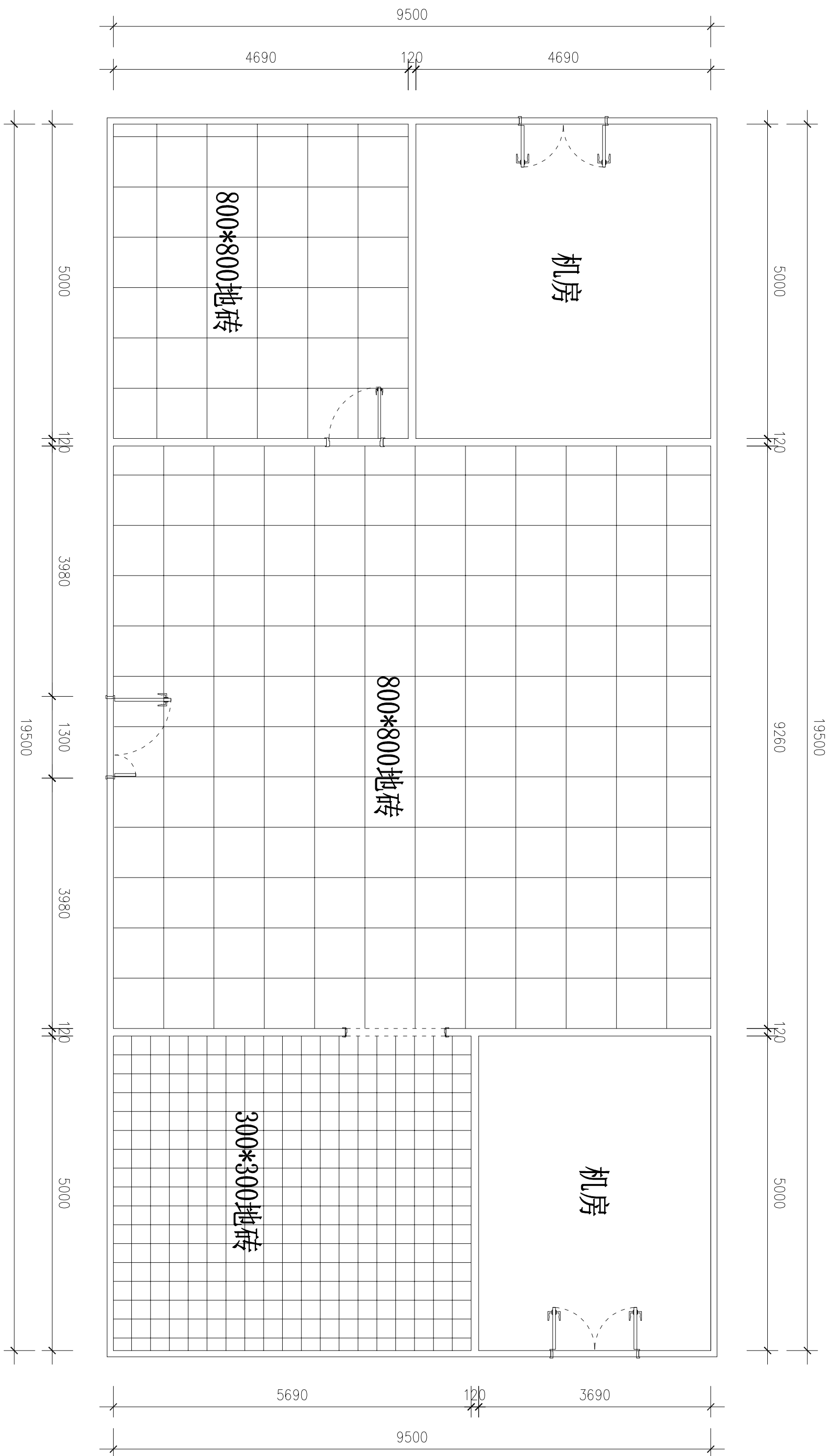
地面-铺贴图
