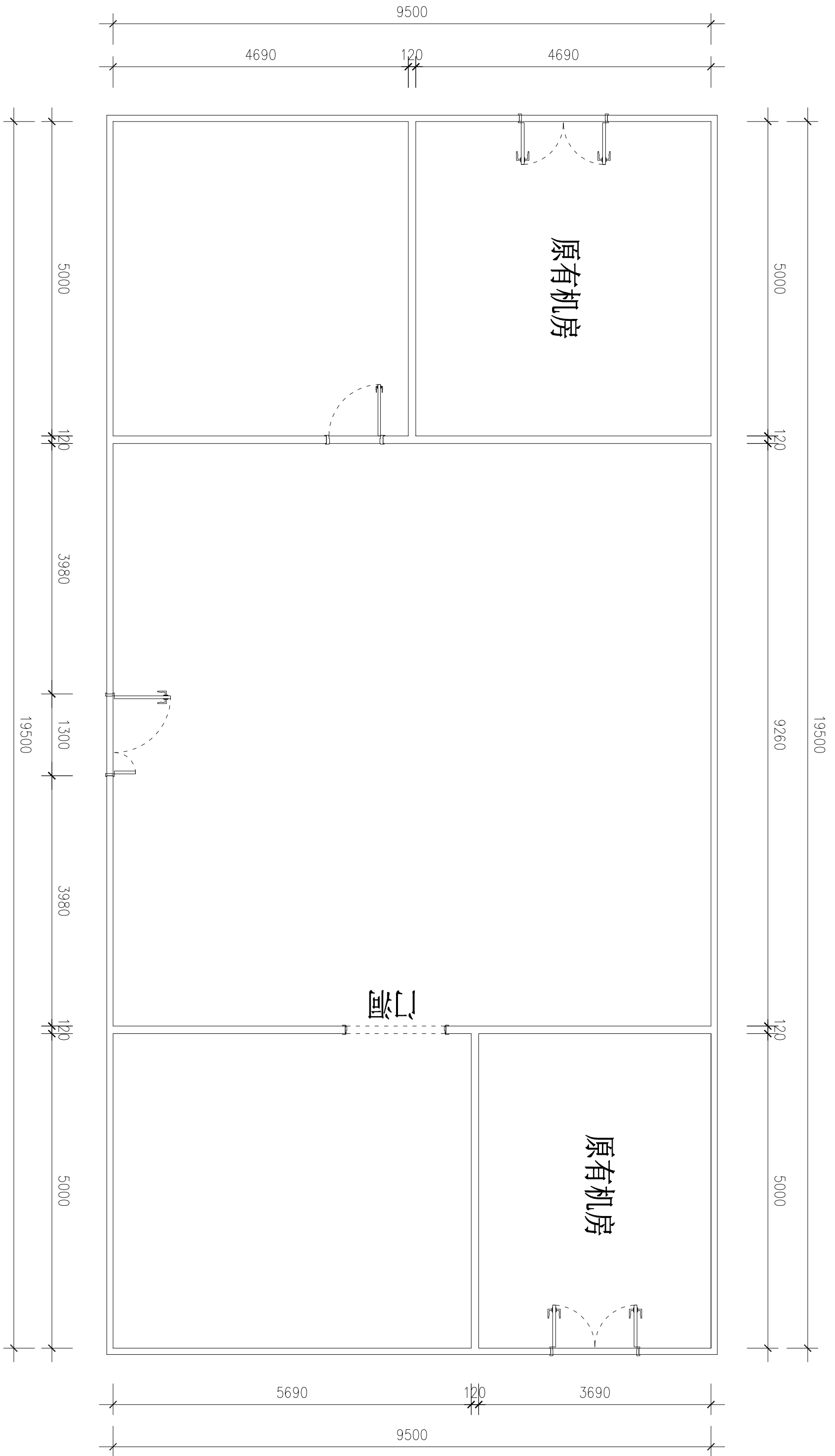
平面布置图
