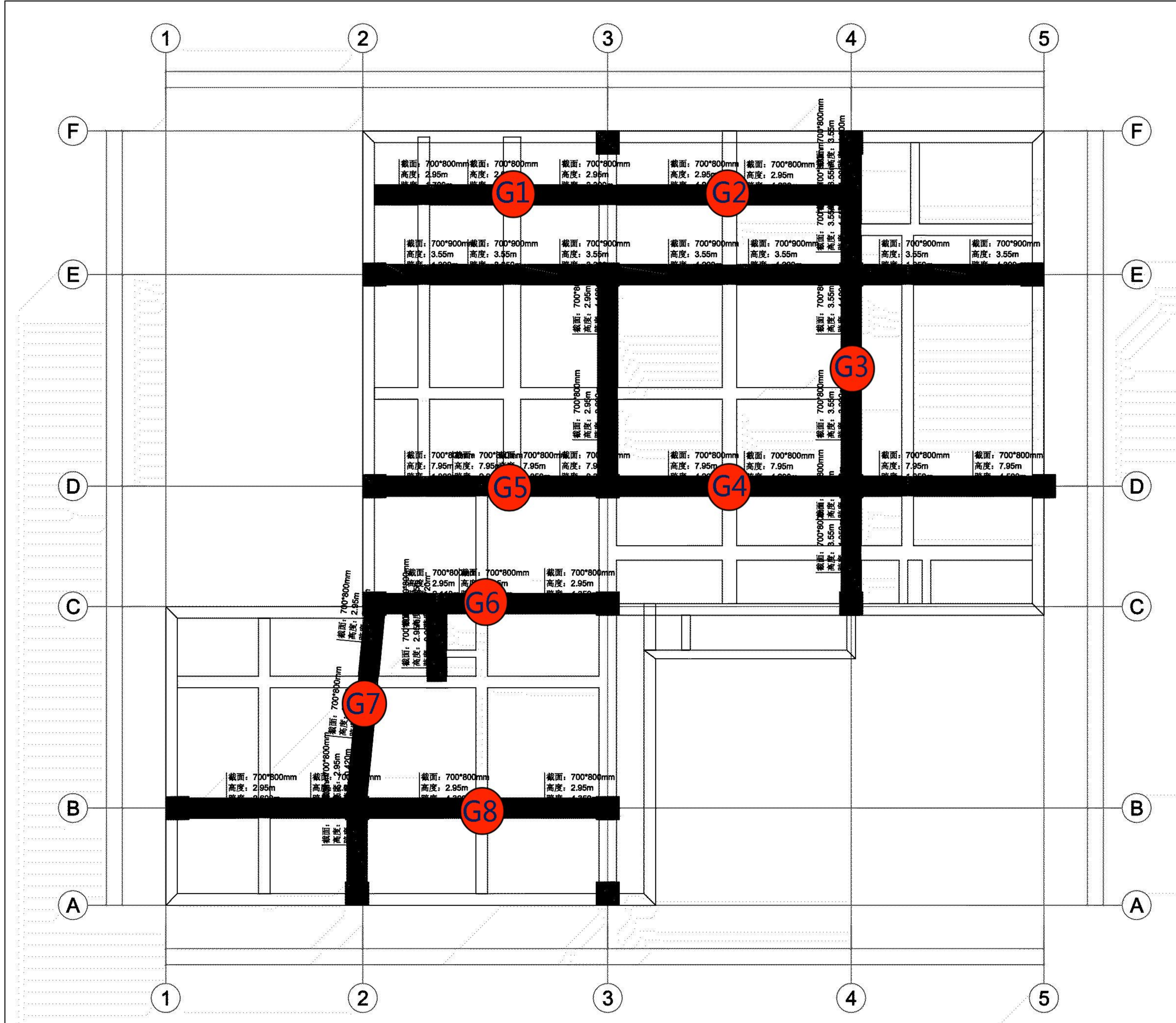
负一层高支模区域分布图
