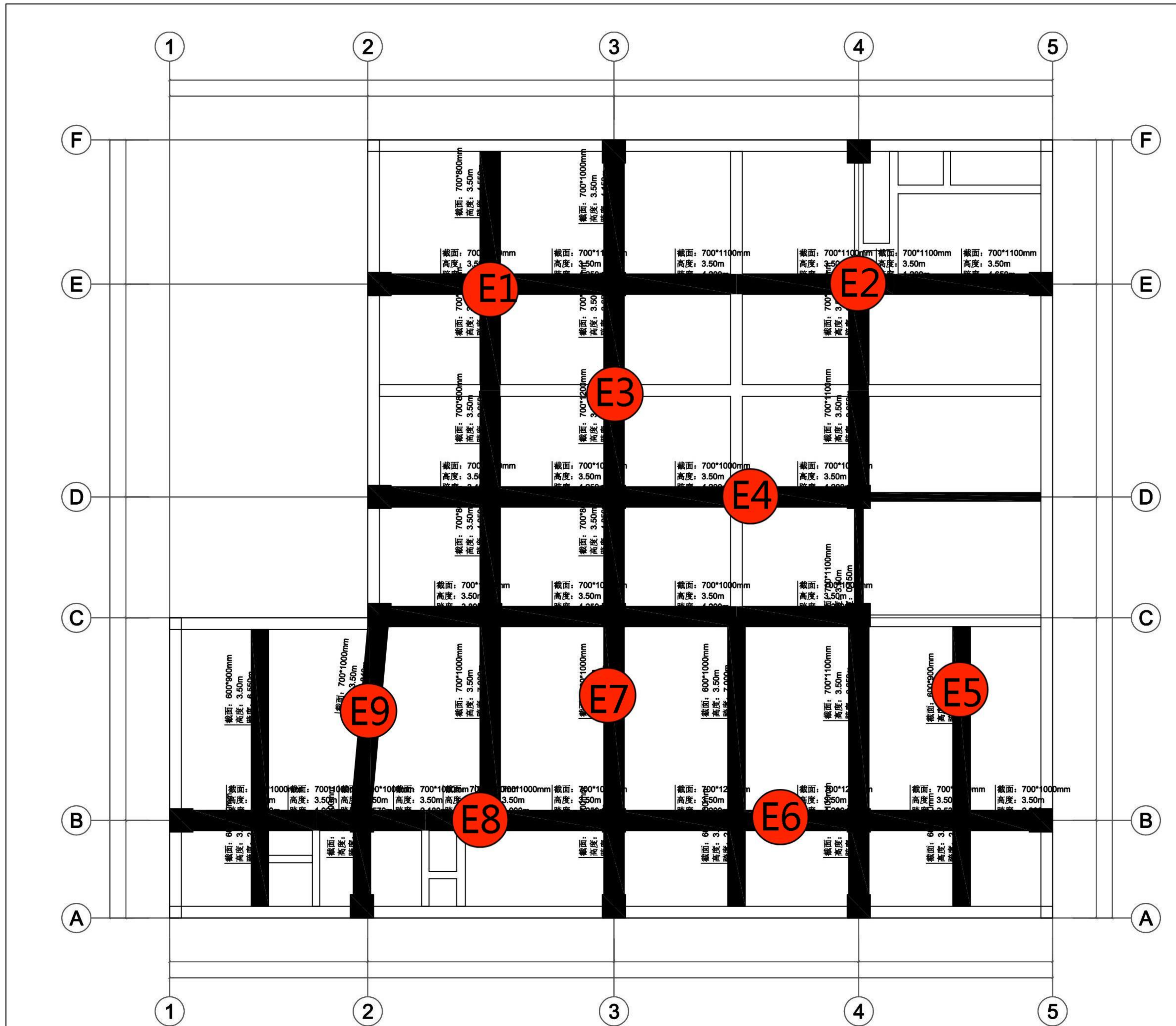
图三 三层高古横区域分布图
